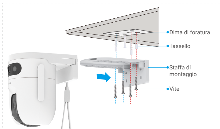
Fig. 1 Montaggio a soffitto
